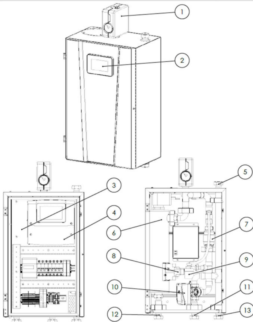
Rysunek 1 – Budowa Hydroboxu HBSP (wersja z pompą wody)
