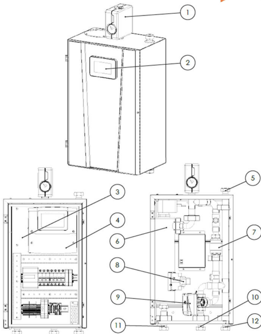
Rysunek 2 – Budowa Hydroboxu HBSB (wersja bez pompy wody)
